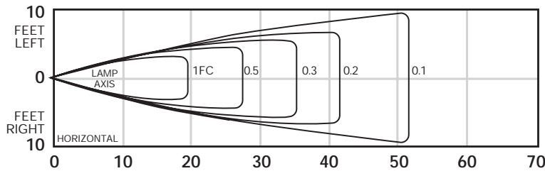
12 Volt Incandescent 12 Watt
